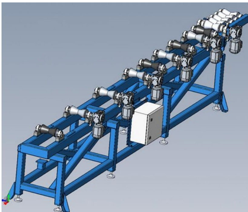
Mesa de Roletes Frontal
